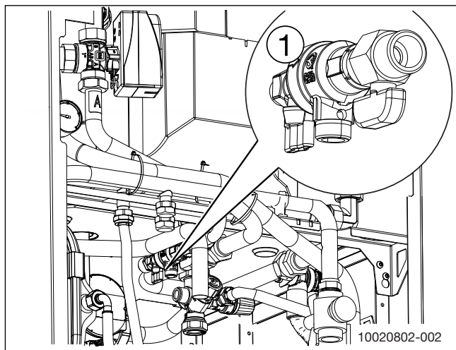
Kuva 6 Lämmityslaitteiston täyttöhana
