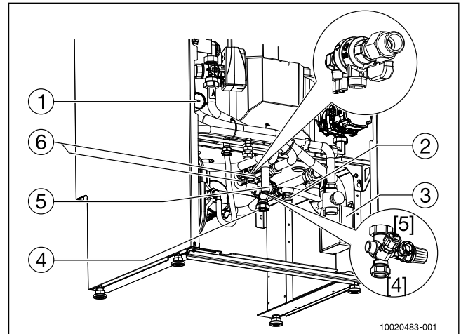
Kuva 4 Liitäntäalue
