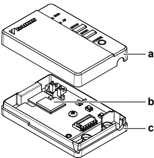
a Yläkotelo b Langattoman LAN-sovittimen piirilevy c Alakotelo
