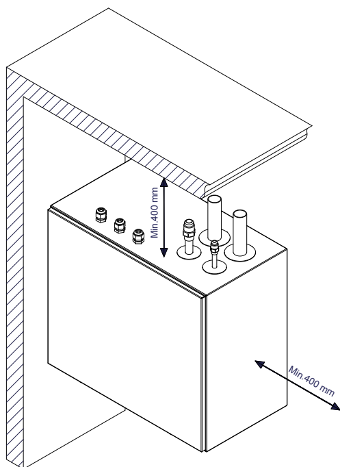
Kuva 9. Suositus nurkka-asennukseen.
