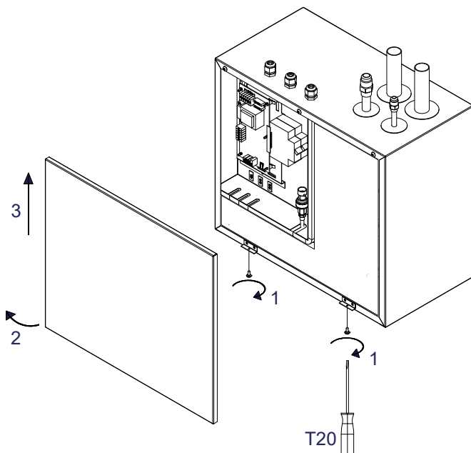
Kuva 10. Etukannen irrottaminen.
