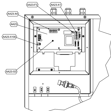
Kuva 4b. Sähkökomponenttien sijainnit tuotteessa R32 kylmäaineella.
