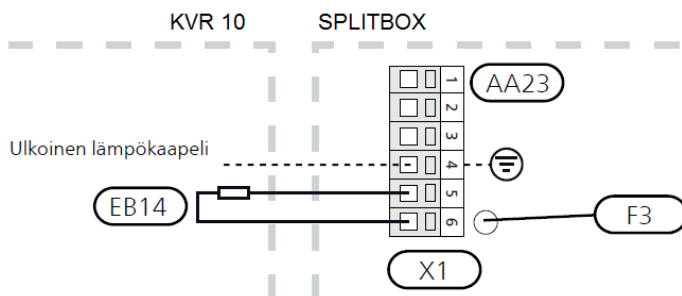
Kuva 13. Ulkoinen lämpökaapeli.
