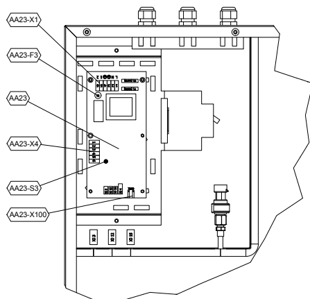
Kuva 4a. Sähkökomponenttien sijainnit tuotteessa R410A kylmäaineella.
