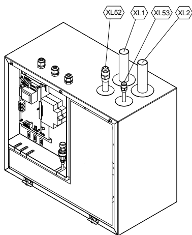
Kuva 11. Putkiliitännät.
