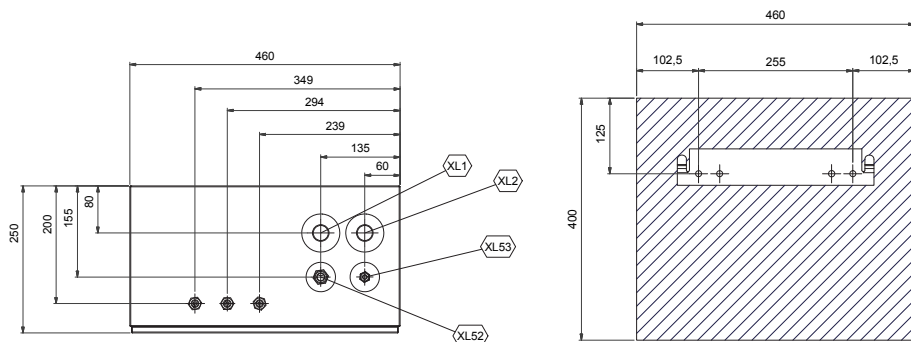
Kuva 5. Mitat.
