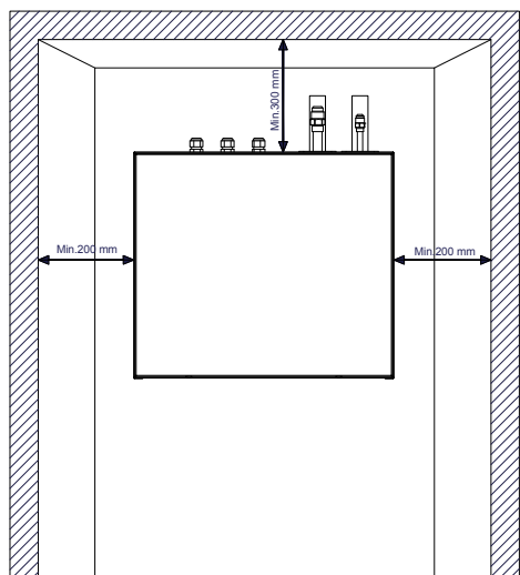
Kuva 8. Suositus seinäasennukseen.
