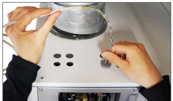
6. Kosketusnäytöltä vedetään kaapeli laitteelle ja yhdistetään piirikortille.
