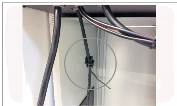
Spacer kappale on kiinnitetty koneessa kiinni olevaan LAN kaapelin(Suurimman peltikuoren alla).
