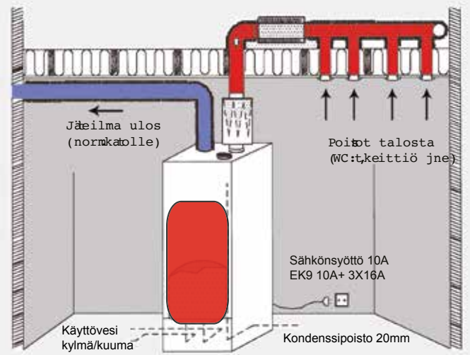
EK9 -mallissa lattia/patterilämmityksen yhteydet pohjassa
